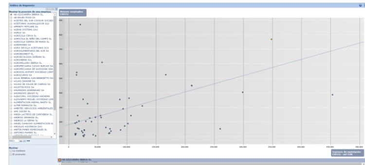
Regresión Lineal
